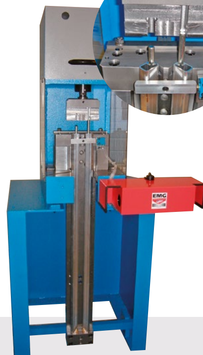
► 6TLP z oprzyrządowaniem do mocowania sworzni i modyfikacją ramy
