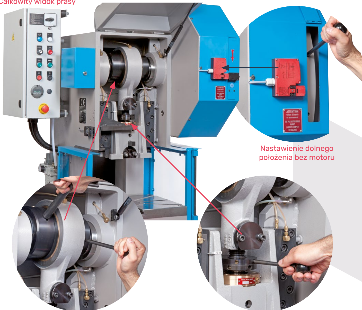
Szybka regulacja suwu
