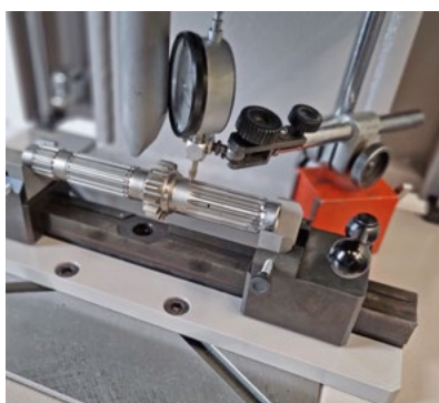
► 6TLP z narzędziem do prostowania wałów
